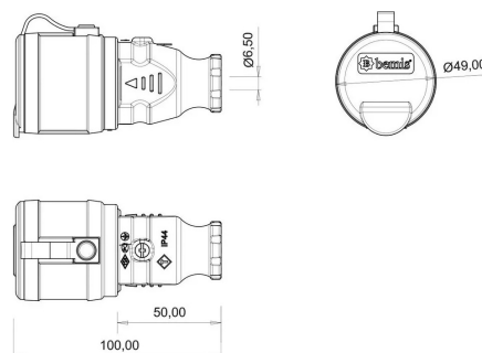
ГАБАРИТНЫЙ ЧЕРТЁЖ
