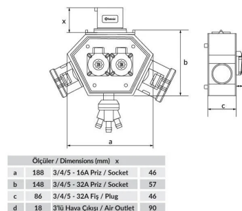
ГАБАРИТНЫЙ ЧЕРТЁЖ
