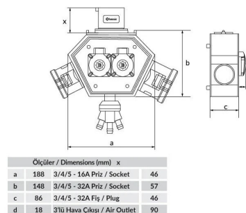
ГАБАРИТНЫЙ ЧЕРТЁЖ
