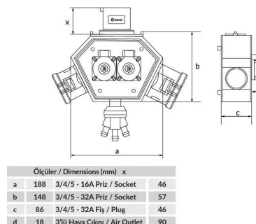
ГАБАРИТНЫЙ ЧЕРТЁЖ
