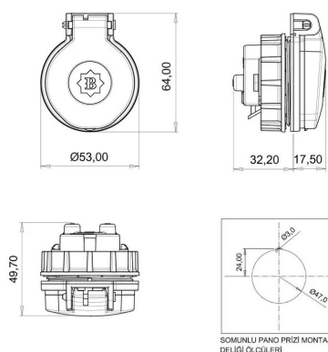
ГАБАРИТНЫЙ ЧЕРТЁЖ
