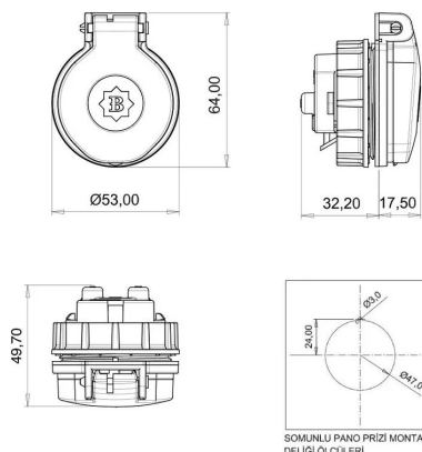
ГАБАРИТНЫЙ ЧЕРТЁЖ
