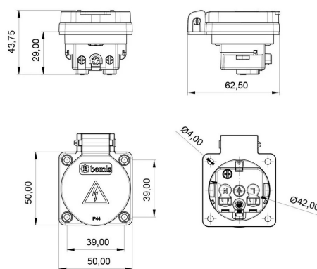
ГАБАРИТНЫЙ ЧЕРТЁЖ
