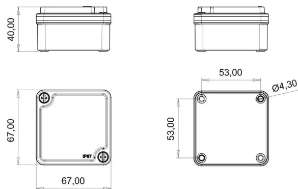
ГАБАРИТНЫЙ ЧЕРТЁЖ
