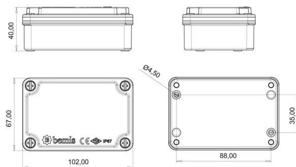
ГАБАРИТНЫЙ ЧЕРТЁЖ
