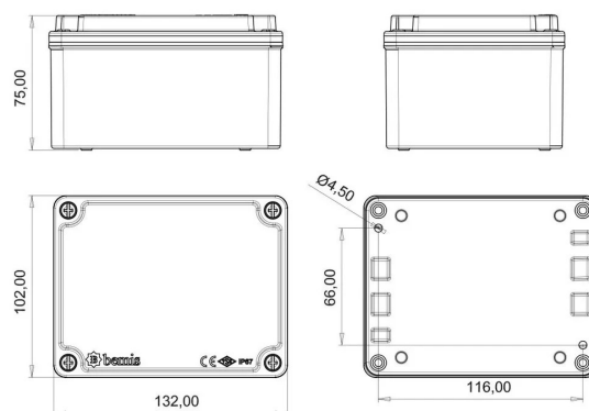
ГАБАРИТНЫЙ ЧЕРТЁЖ
