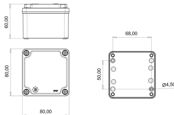
ГАБАРИТНЫЙ ЧЕРТЁЖ
