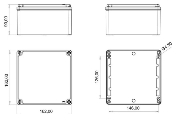
ГАБАРИТНЫЙ ЧЕРТЁЖ
