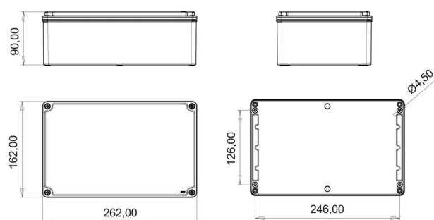
ГАБАРИТНЫЙ ЧЕРТЁЖ
