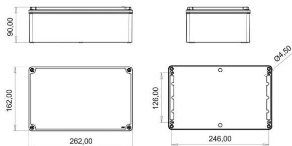
ГАБАРИТНЫЙ ЧЕРТЁЖ
