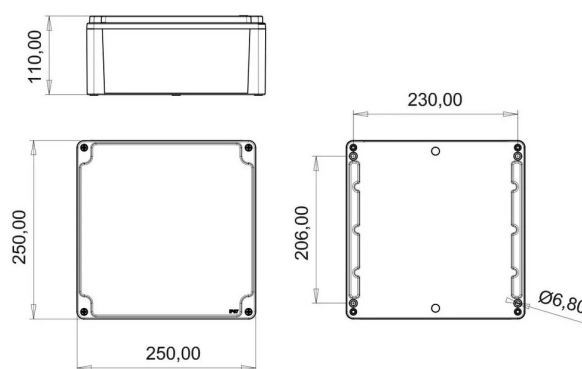
ГАБАРИТНЫЙ ЧЕРТЁЖ
