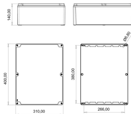
ГАБАРИТНЫЙ ЧЕРТЁЖ
