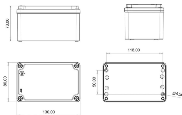
ГАБАРИТНЫЙ ЧЕРТЁЖ
