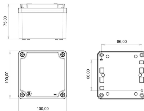
ГАБАРИТНЫЙ ЧЕРТЁЖ
