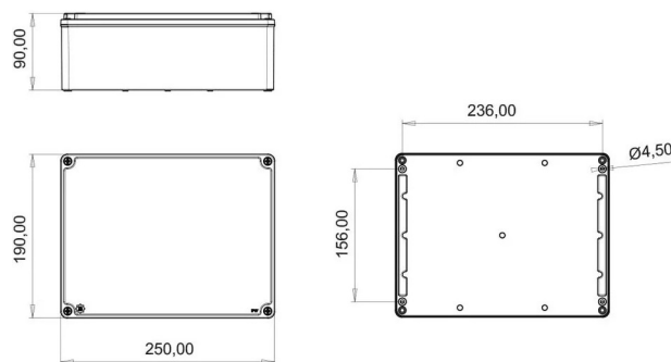
ГАБАРИТНЫЙ ЧЕРТЁЖ
