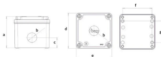
ГАБАРИТНЫЙ ЧЕРТЁЖ
