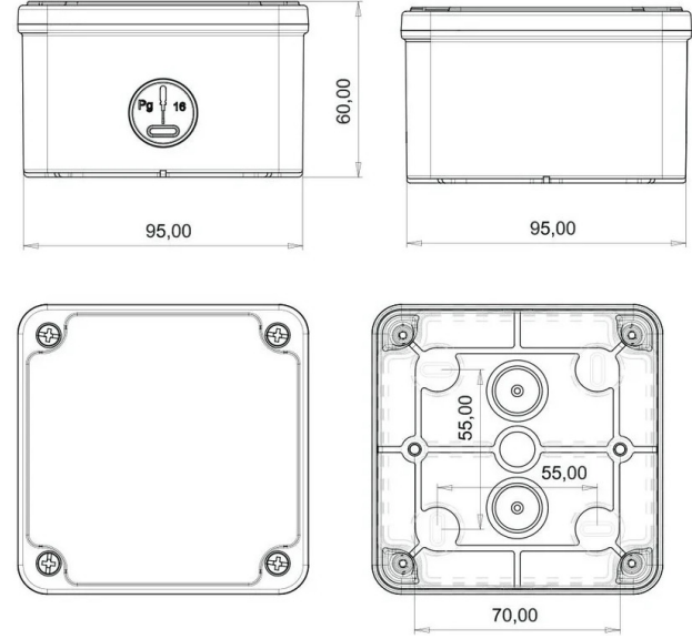
TEKNİK RESİM
