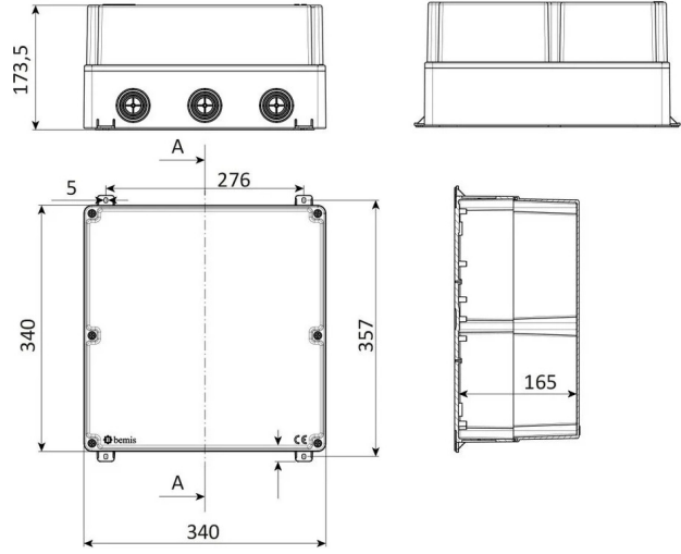
TEKNİK RESİM
