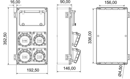
TEKNİK RESİM
