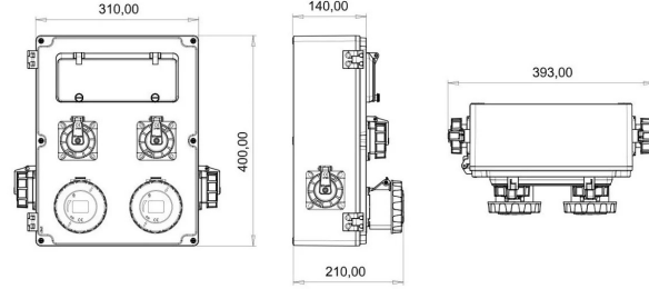
TEKNİK RESİM
