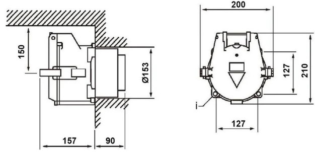
TEKNİK RESİM
