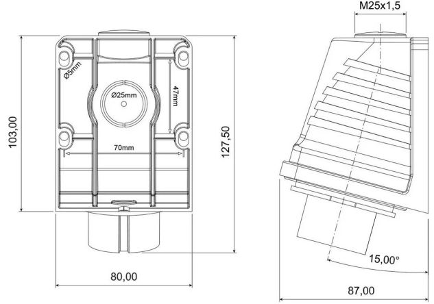
TEKNİK RESİM
