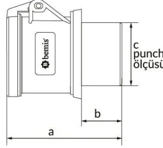
TEKNİK RESİM
