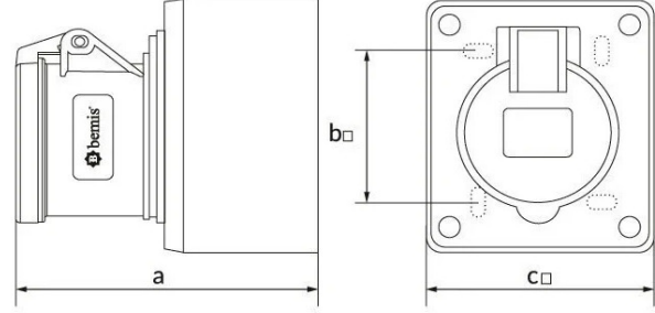
Ölçüler / Dimensions (mm)
