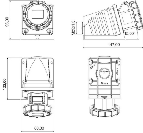
TEKNİK RESİM
