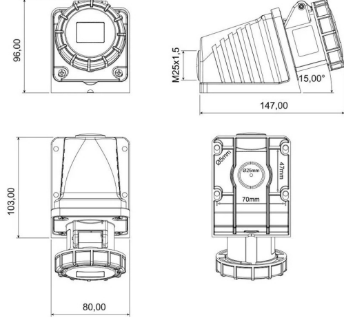
TEKNİK RESİM
