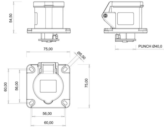
TEKNİK RESİM
