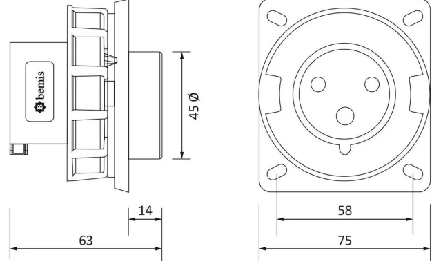
TEKNİK RESİM
