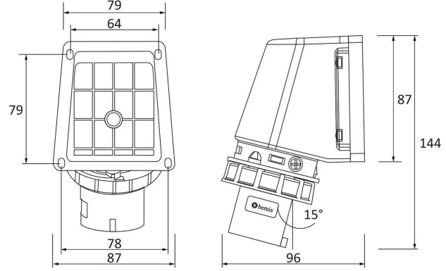
TEKNİK RESİM
