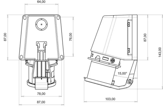
TEKNİK RESİM
