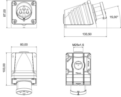
TEKNİK RESİM
