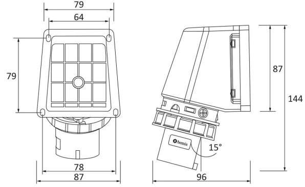
TEKNİK RESİM
