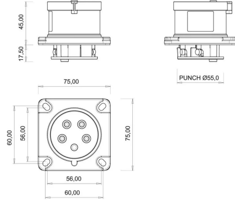
TEKNİK RESİM
