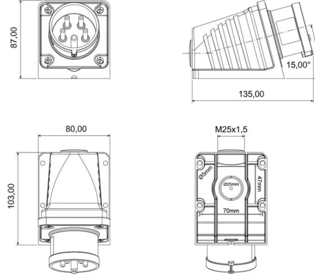
TEKNİK RESİM
