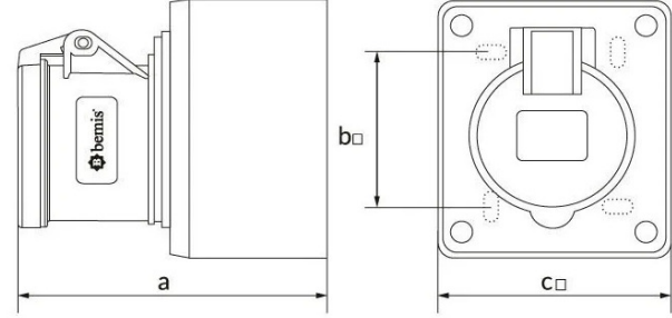
Ölçüler / Dimensions (mm)
