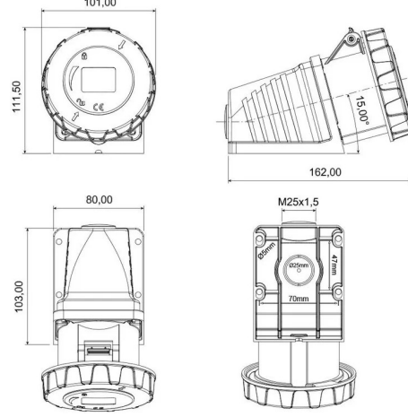
TEKNİK RESİM
