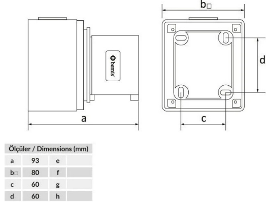
TEKNİK RESİM
