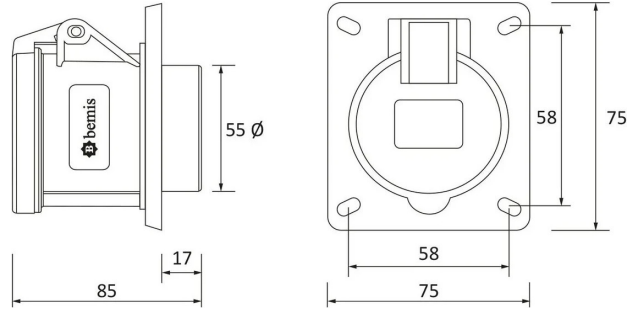
TEKNİK RESİM
