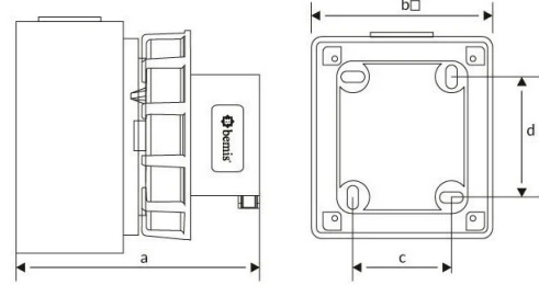
TEKNİK RESİM
