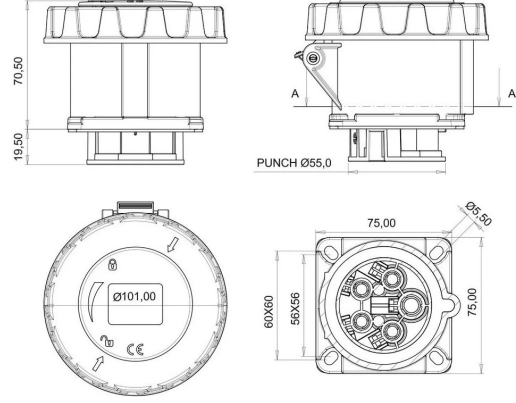
TEKNİK RESİM
