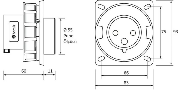
TEKNİK RESİM
