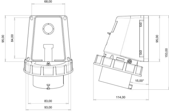
TEKNİK RESİM
