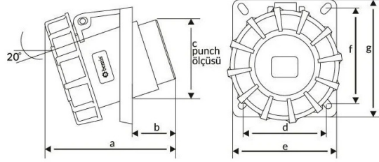
TEKNİK RESİM
