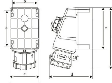
Ölçüler / Dimensions (mm)
