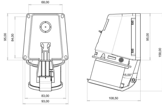
TEKNİK RESİM
