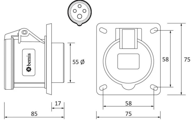
TEKNİK RESİM
